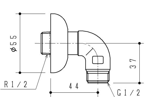
リモデル壁給水用エルボ
