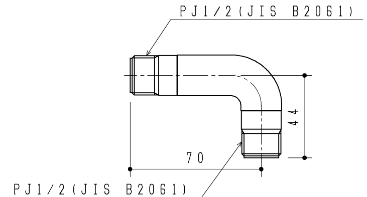
リモデル壁給水用エルボ
