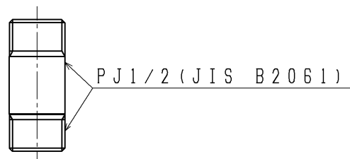
リモデル床給水用ニップル
